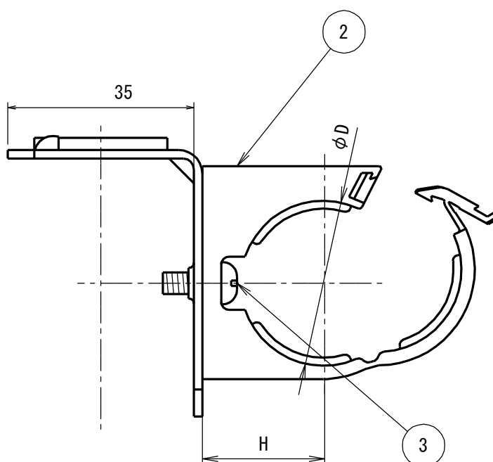
図はLSFBM-25を示す。
